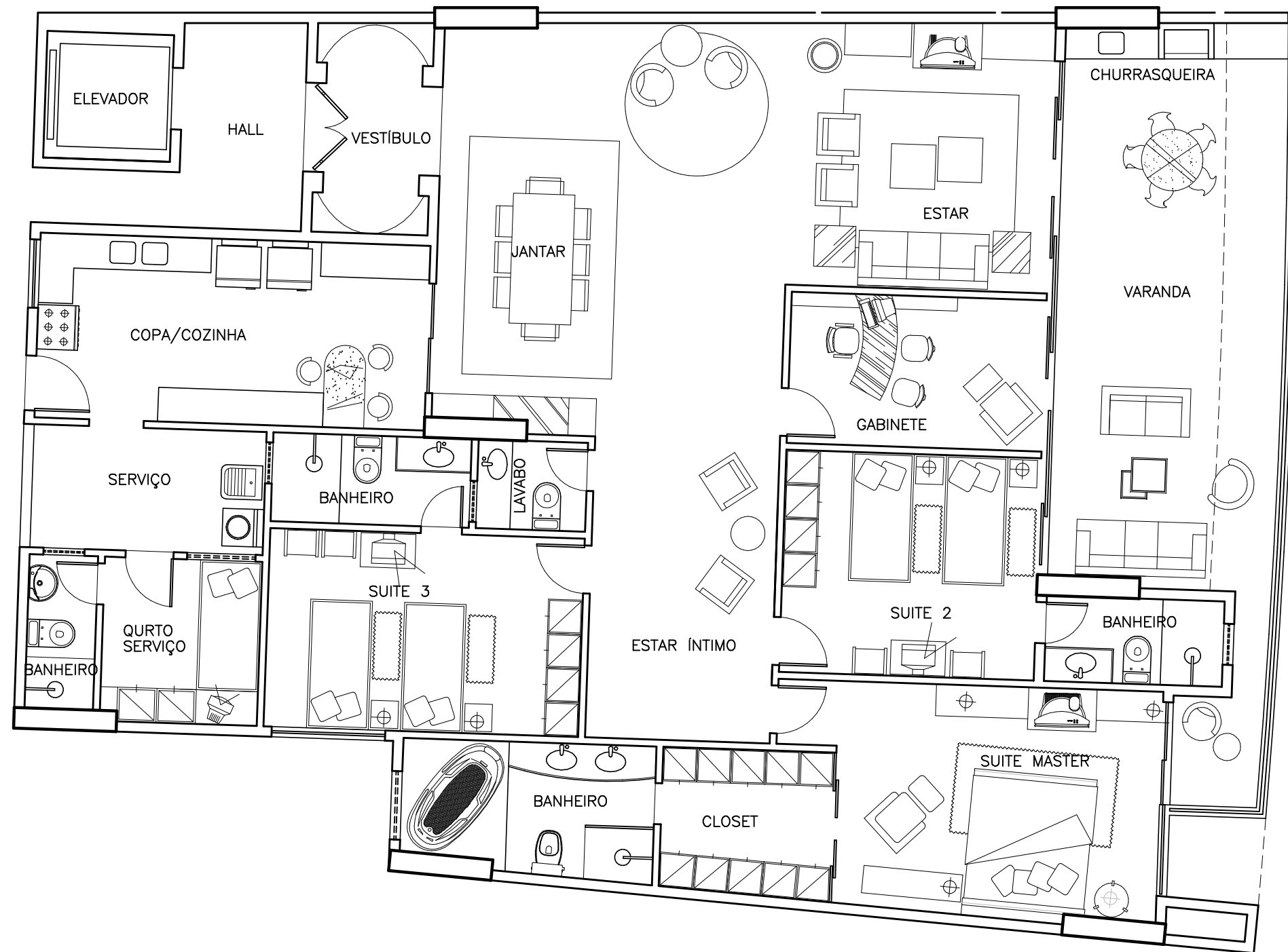
01 APTO DO CANTO ESCALA 1/75
